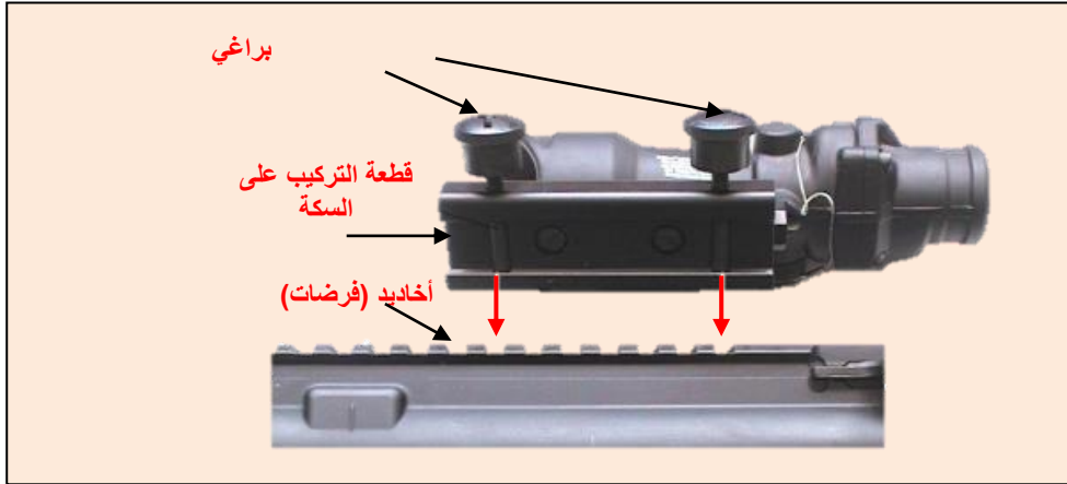
الشكل (112) تركيب منظار البندقية القتالي
