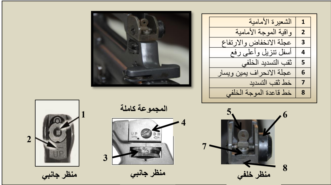
الشكل (14) التصفير اليدوي لموجهات الرماية للبندقية إم 16 أ2
