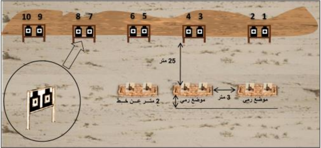
الشكل (15) ميدان تجميع الرماية على مسافة 25 متراً
