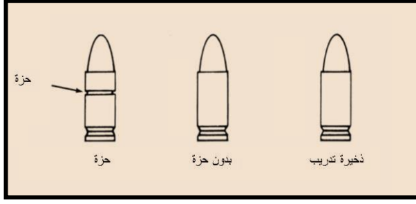
الشكل (92) ذخيرة مسدس كراكال عيار 9 ملم
