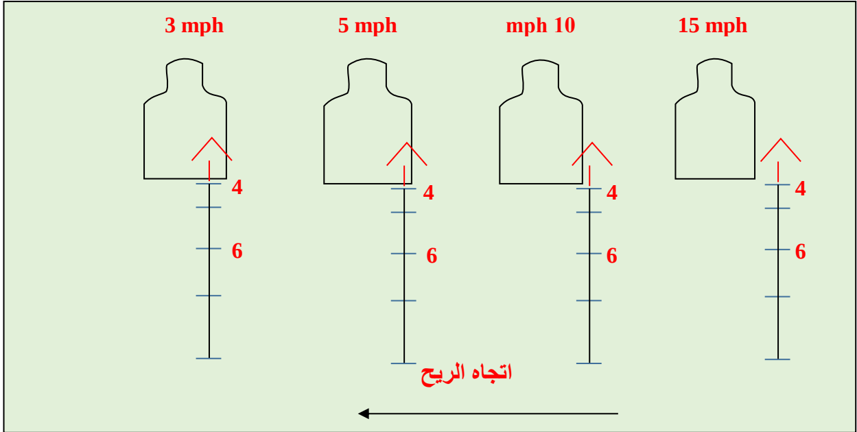
الشكل (66) تضبيط موجه الاتجاه على مسافة 300 م
