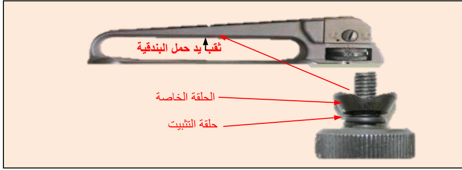
الشكل (116) وضع مجموعة البرغي
