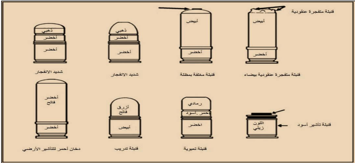
الشكل (94) ذخيرة قاذف القنابل عيار 40 ملم
