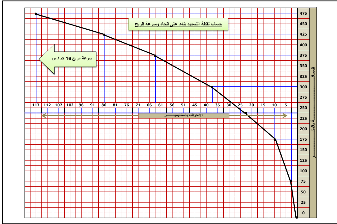
الشكل (40) حساب نقطة التسديد التي تم تضبيطها بناءً على سرعة الرياح
