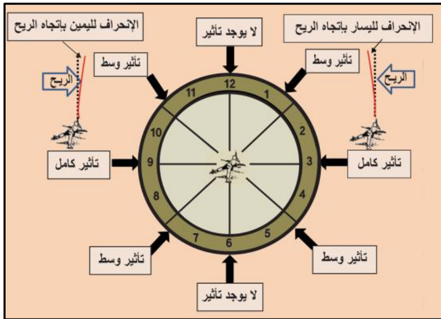
الشكل (38) تحديد مقدار قوة الريح باستخدام طريقة الساعة
