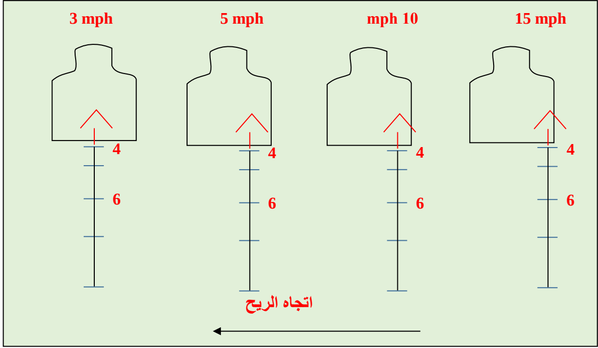
الشكل (65) تضبيط موجه الاتجاه على مسافة 200 م
