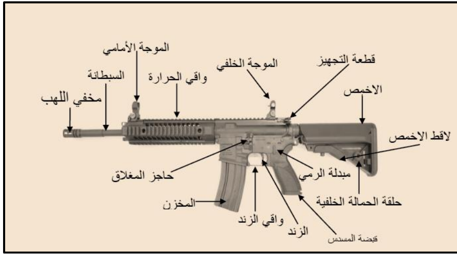
الشكل (90) الوصف العام للبندقية (سلطان)
